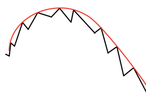
صدف نزولی
