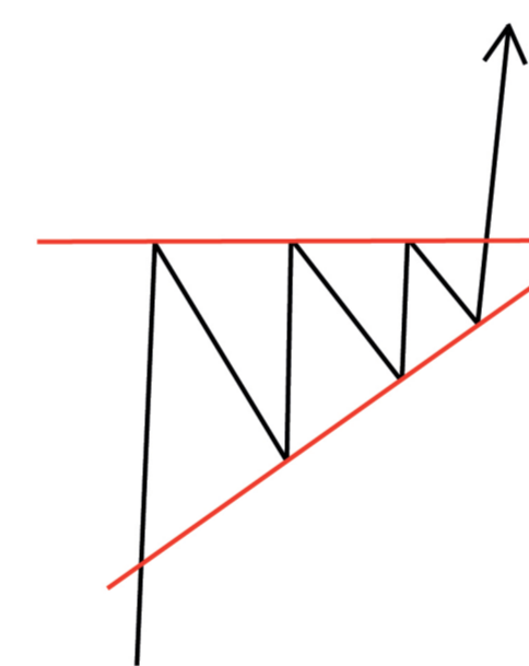
مثلث صعودی
