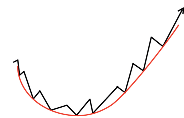
صدف صعودی
