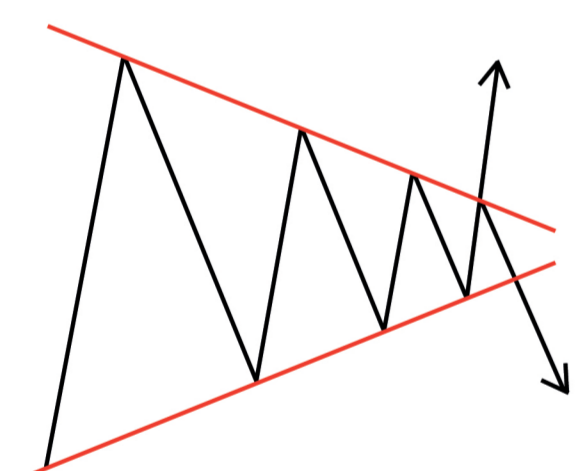
مثلث بسته
