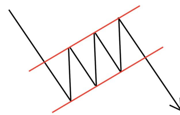
پرچم نزولی
