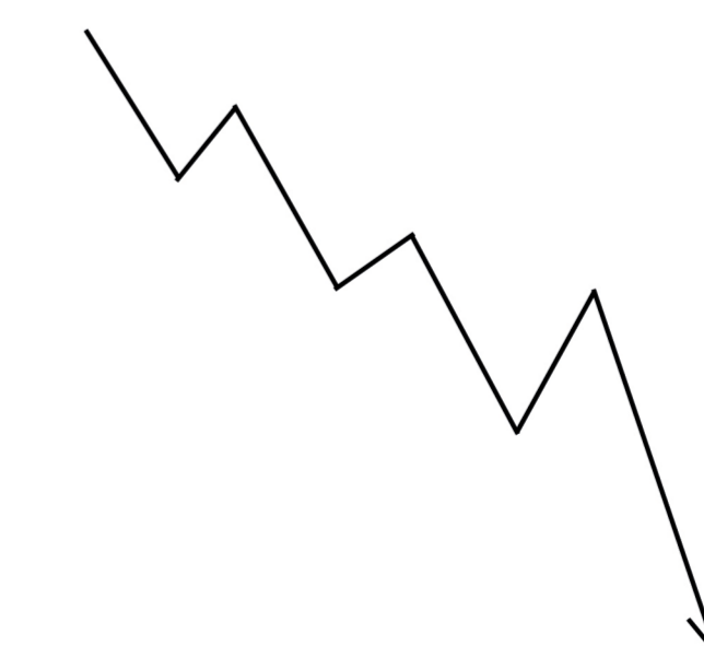
روند نزولی
