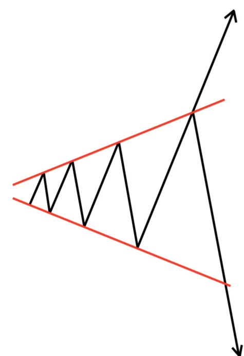
مثلث باز
