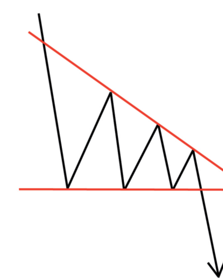
مثلث نزولی
