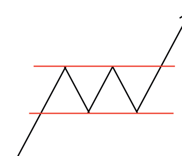
مستطیل صعودی
