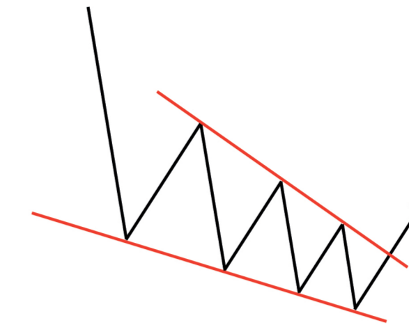
کنج صعودی
